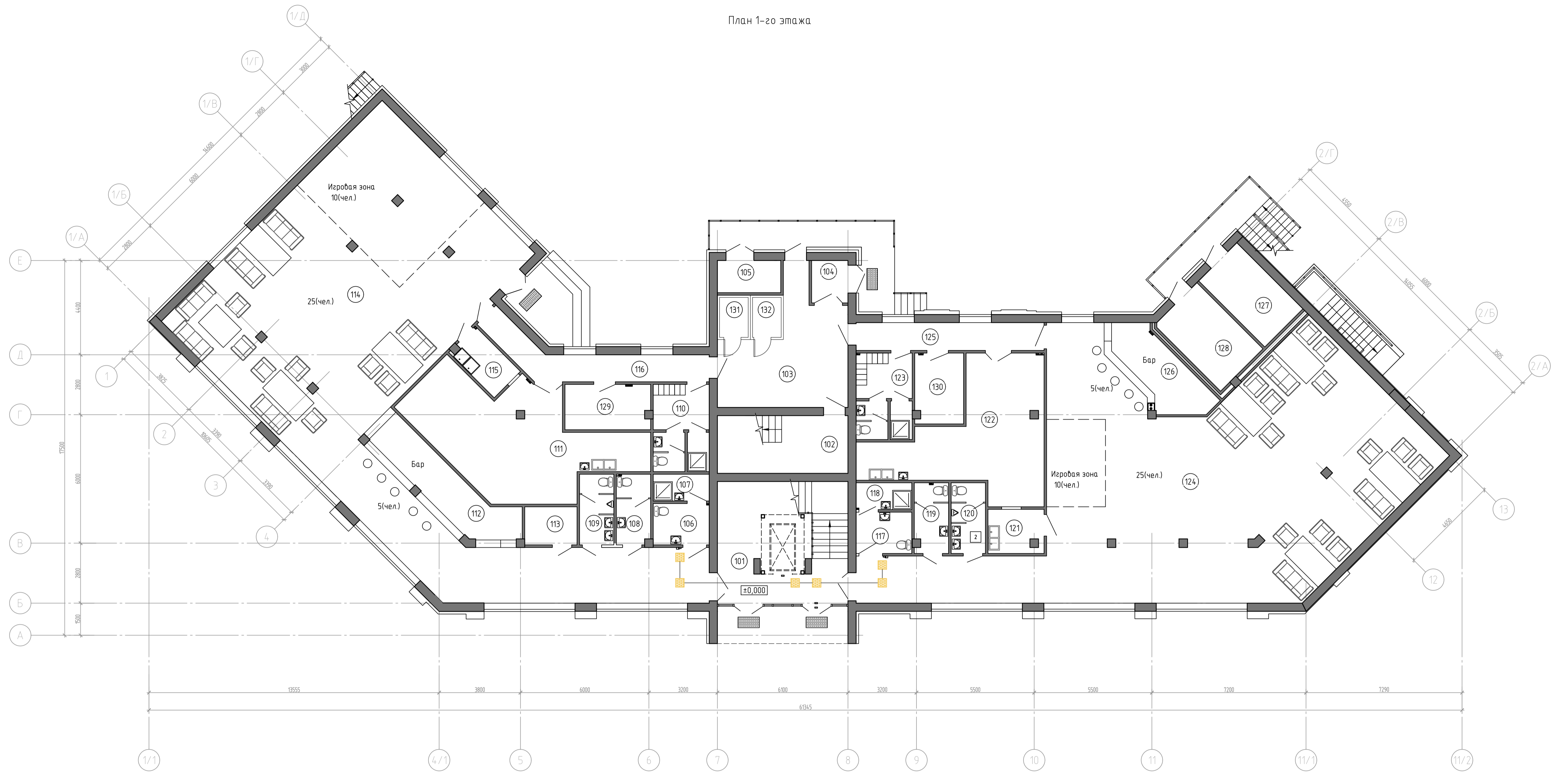
ЭКСПЛИКАЦИЯ ПОМЕЩЕНИЙ (1-ый этаж)
